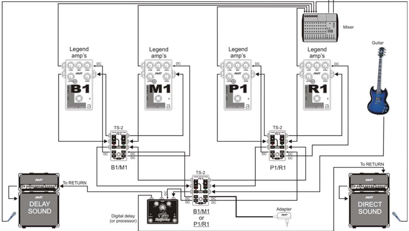
Legend-R1 Block-diagram. Legend-R1 Блок-схема.
