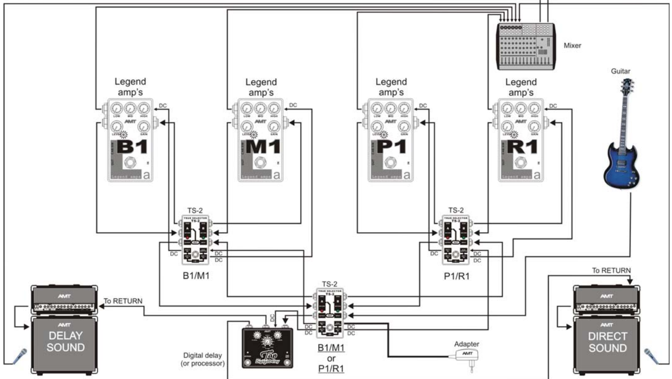
Legend-M1 Block-diagram. Legend-M1 Блок-схема.
