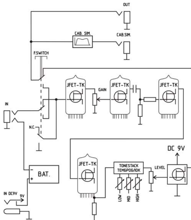
Legend-M1 Block-diagram. Legend-M1 Блок-схема.
